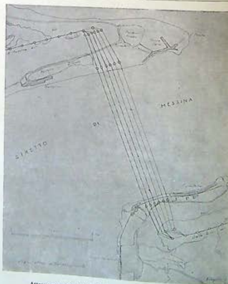
Attraversamento aereo dello Stretto di Messina (planimetria)
