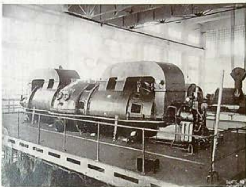
Centrale termoelettrica di Porto Empedocle - il nuovo tubo alternatore da 10.000 KW.
