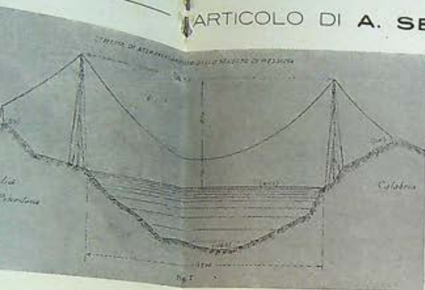
Progetto di attraversamento aereo dello Stretto.
