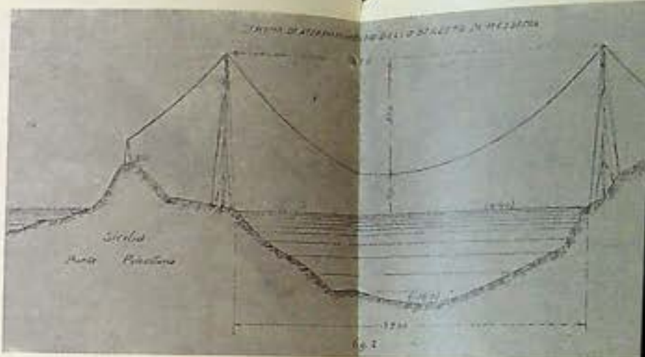
Progetto di attraversamento aereo dello Stretto
